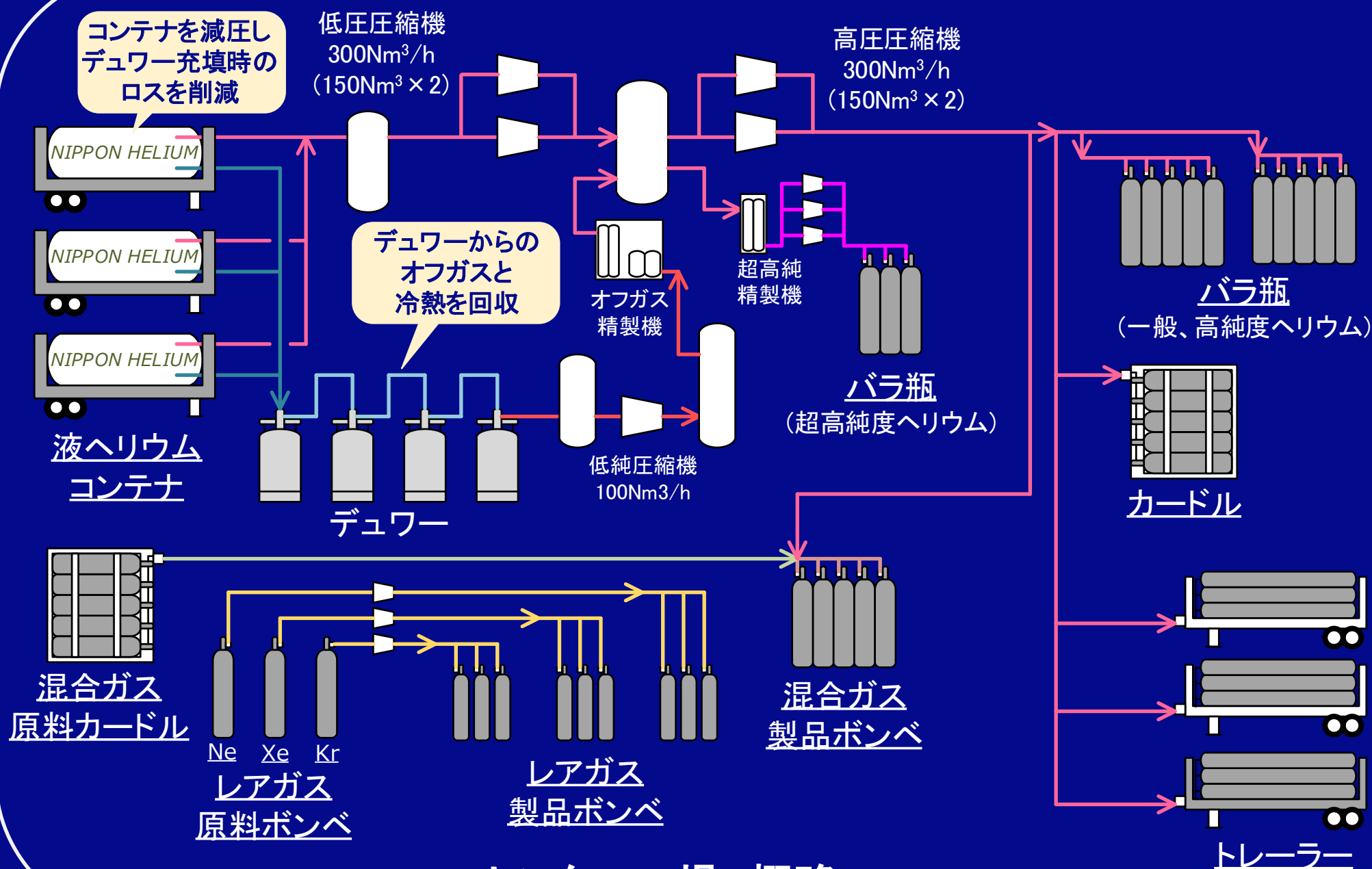
センター工場 概略フロー
